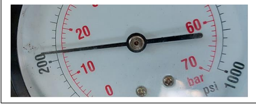
Cilindro # 1 valor de compresión 210 psi, 15 bar
